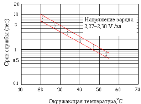
Зависимость срока службы от окружающей температуры
